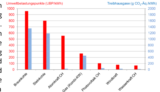
Umweltbelastungspunkte verschiedener Arten der Stromerzeugung. Quelle: E2 Management Consulting AG,
